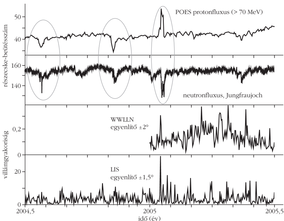
8. ábra. Műholdon mért protonfluxus (legfölel), a Jungfraujoch (Svájc) földi állomás neutronfluxusa (alatta), illetve egy WWLLN és LIS műholdas adatbázisból kinyert villámgyakoriság időfejlődése. Az első két ellipszis Forbush-eseményeket, a harmadik a Napból érkező 2005. január 15-i protonzáport jelöli, részletek a szövegben.
